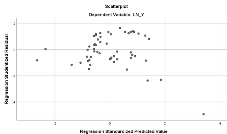
Gambar 3. Grafik Scatterplot
