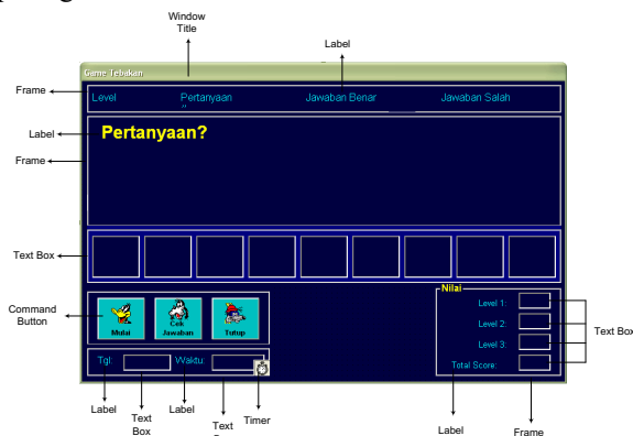
Gambar 9. Rancangan Dialog Game Tebakan
