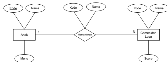
Gambar 15. ERD
